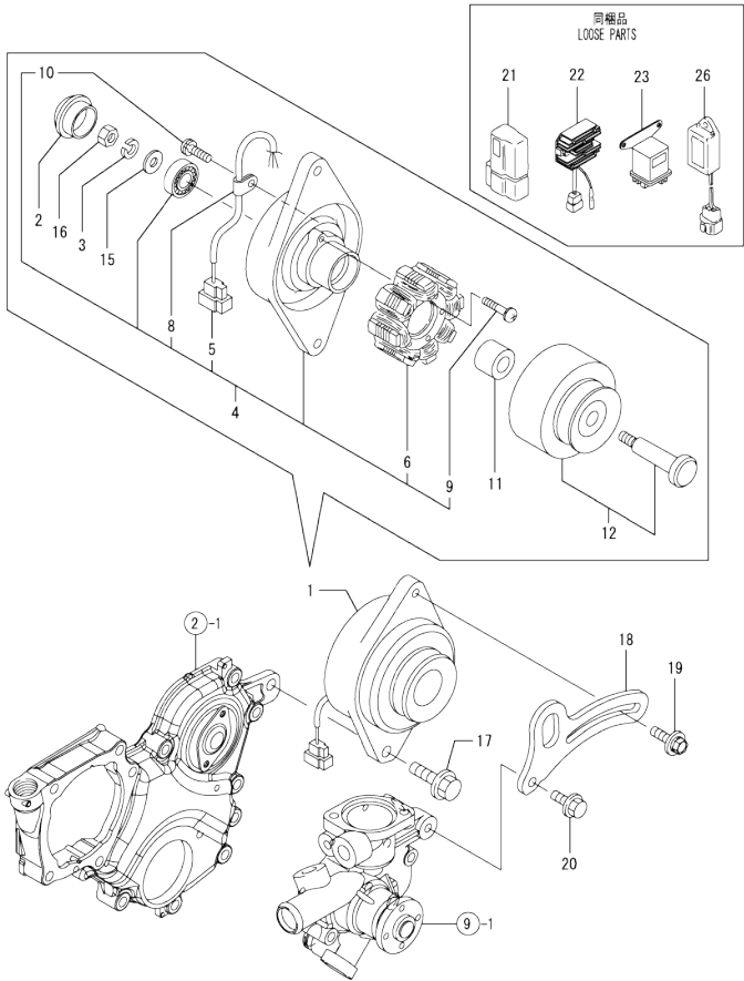
Fig.15. GENERATOR
